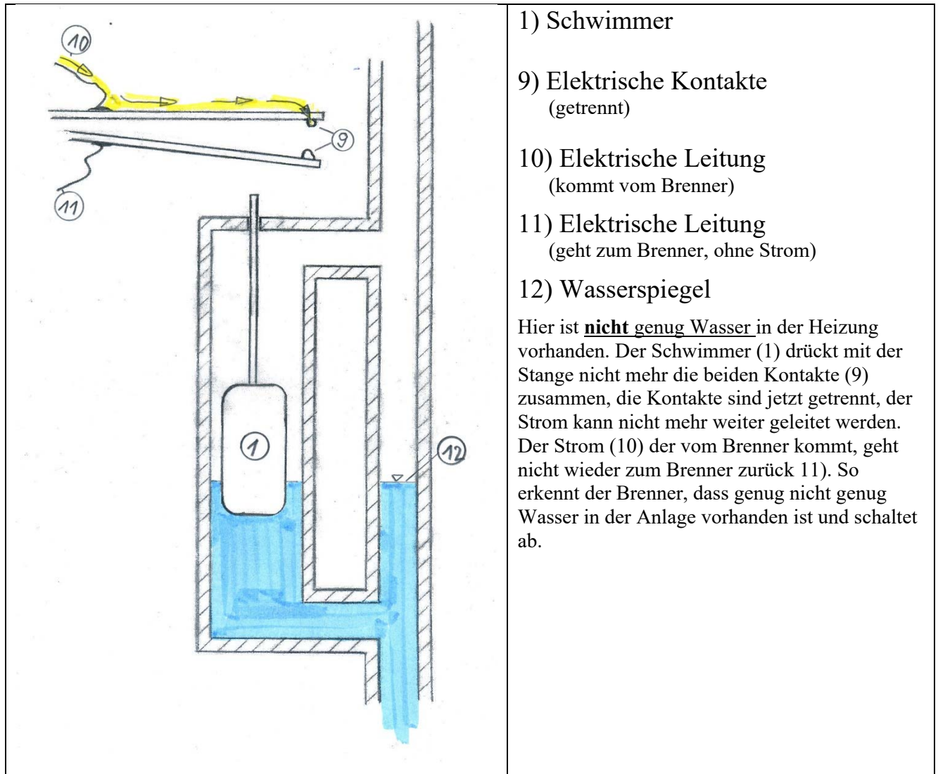
Bild 3: Wasser-Mangelsicherung, elektrische Kontakte getrennt
