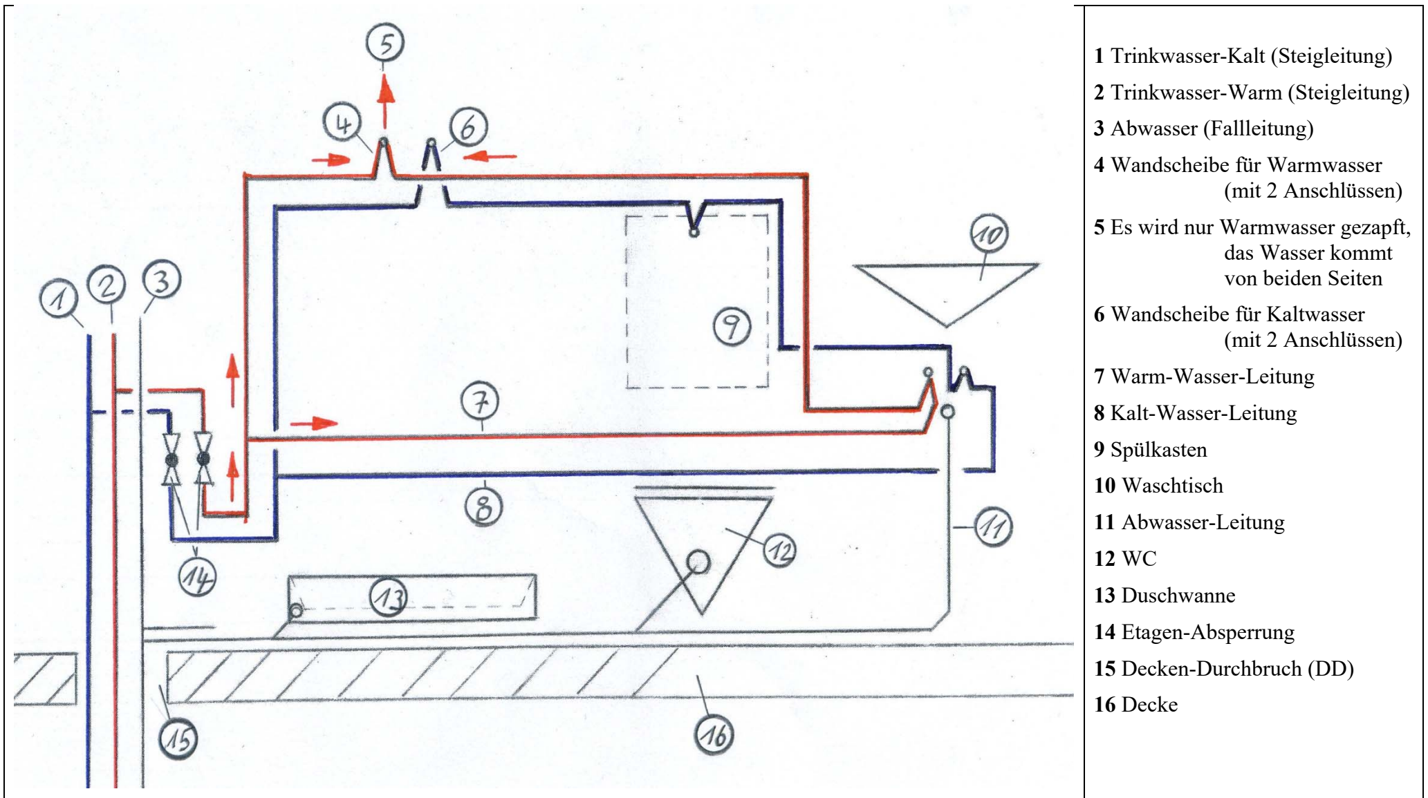
Bild 3: Strangenschema der Bad-Installation: Ringleitungs-System. Nur die senkrechten* Maße sind maßstabsgetreu! (*vertikal, lotrecht)
